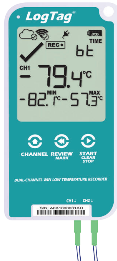
UTREL30-WIFI
